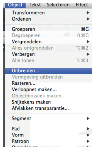
afbeelding 3.1 - Object > Uitbreiden...
